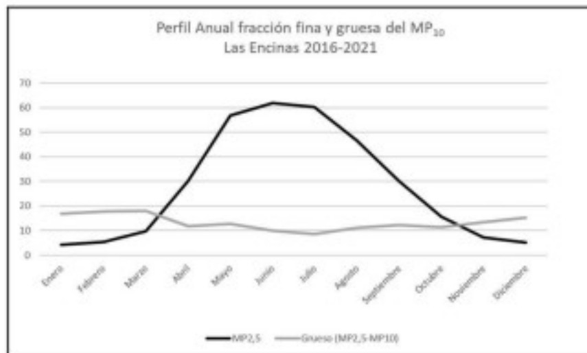
Gráfico N° 5. Perfil anual del MP 2,5 y MP 2,5-10
